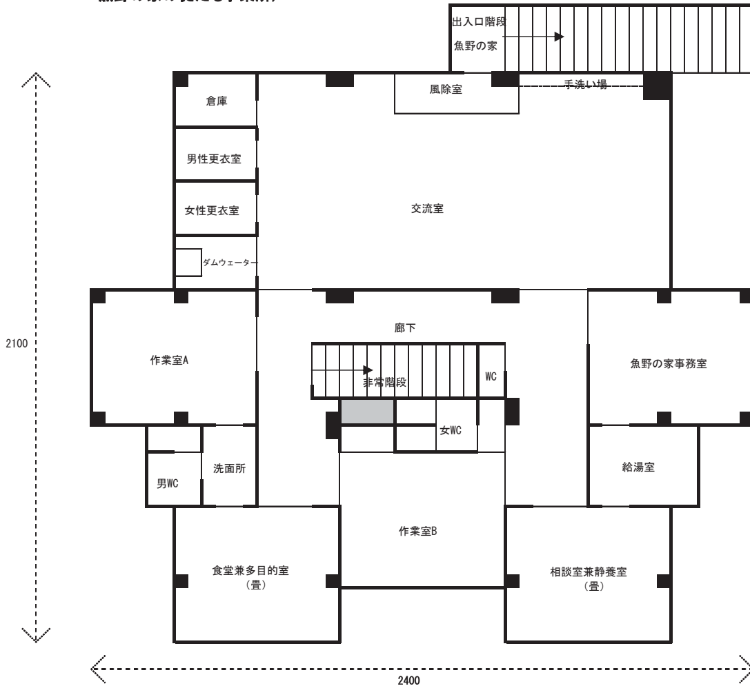
魚野の家うらさ2階平面図 魚野の家の従たる事業所
